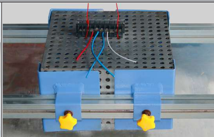
Blocco di connessione durante il test
