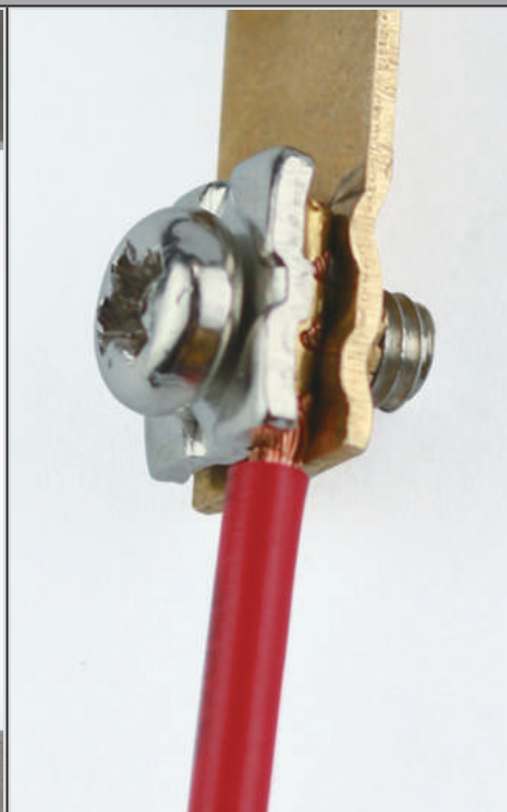
Dettaglio terminale
