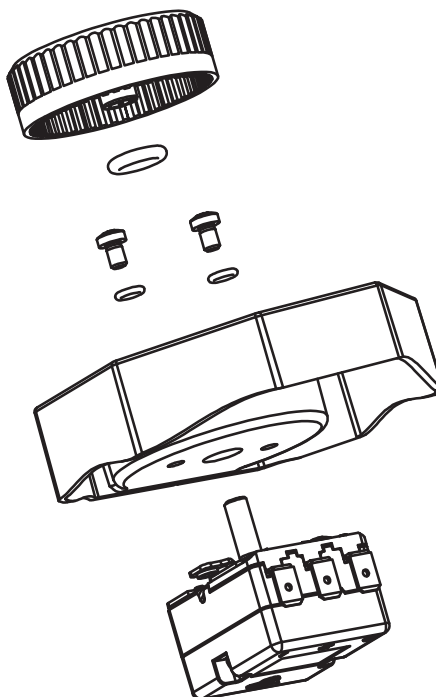
Alloggiamento con manopola termostatica esterna IP69K
