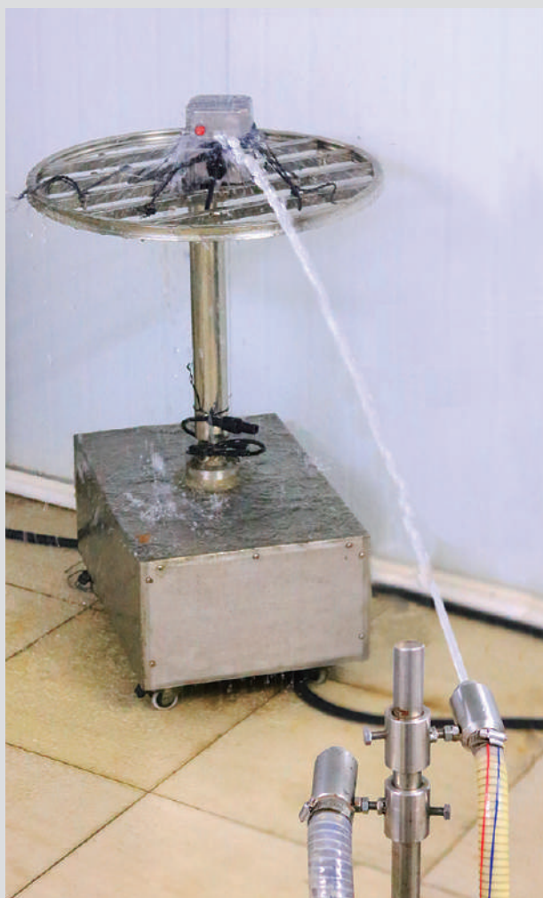
Test IPx5
