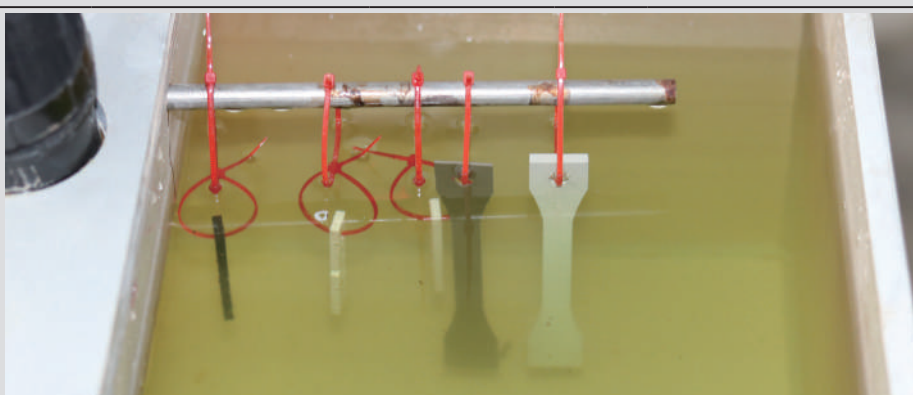
Posizione del campione all'interno del bagno
